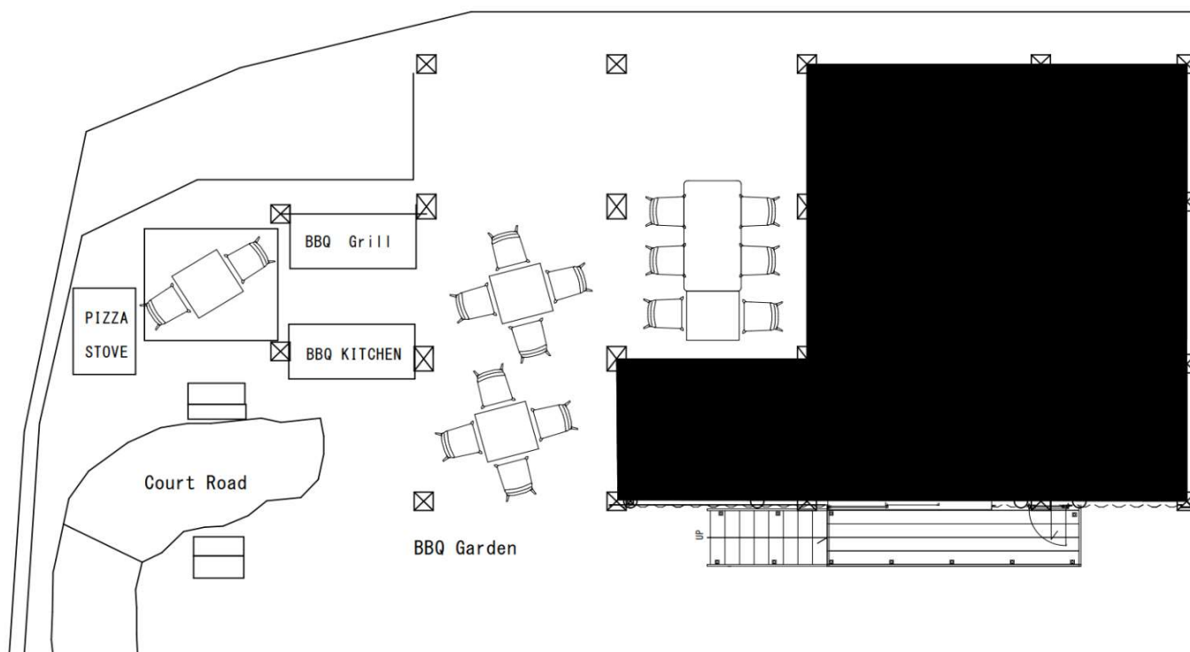
■1F 平面図(BBQ GARDEN)
